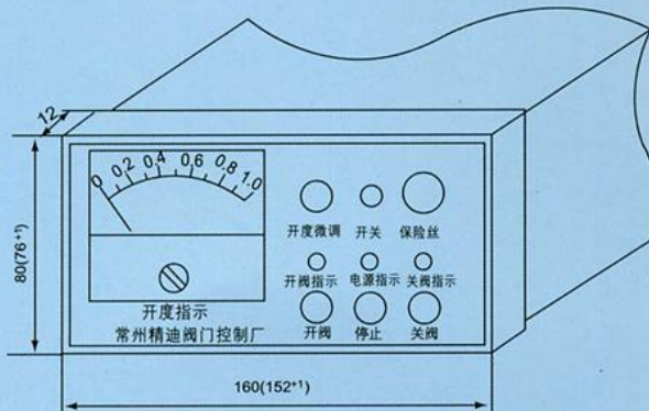
DKX-G型控制箱外形尺寸 (括号内数据为开孔尺寸)
