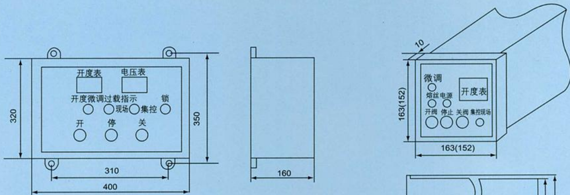
DKX-G型控制箱外形尺寸: 长X宽X高: 400X320X160mm
